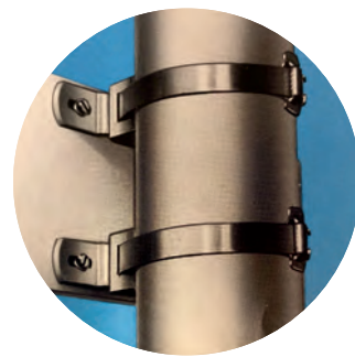
Mittelbefestigung an Masten
